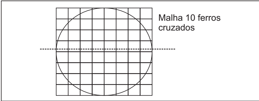
Figura 8 – Estrutura da Malha de Ferro ¼' do Fundo da Cisterna
